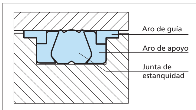
Figura 40 Junta compacta DBM
