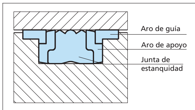
Figura 39 Junta compacta D-A-S, tipo B
